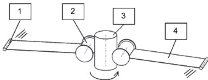
Рис. 1. Двухлопастная тонкопленочная космическая конструкция, стабилизированная вращением:
